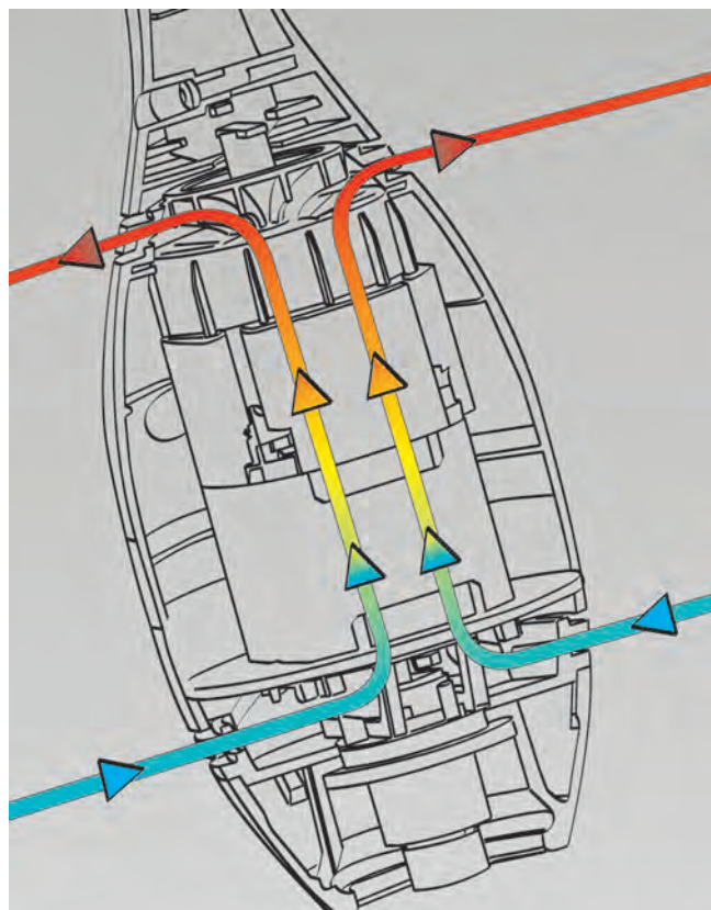
Luftkühlsystem
